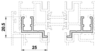
Adjustable Jamb
