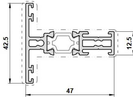
Door Transom
